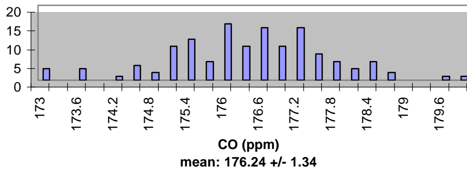
HH T CO
