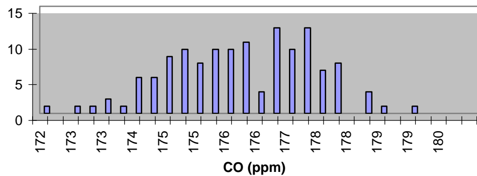
HH S CO
