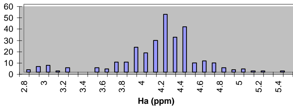
HH Y CO
