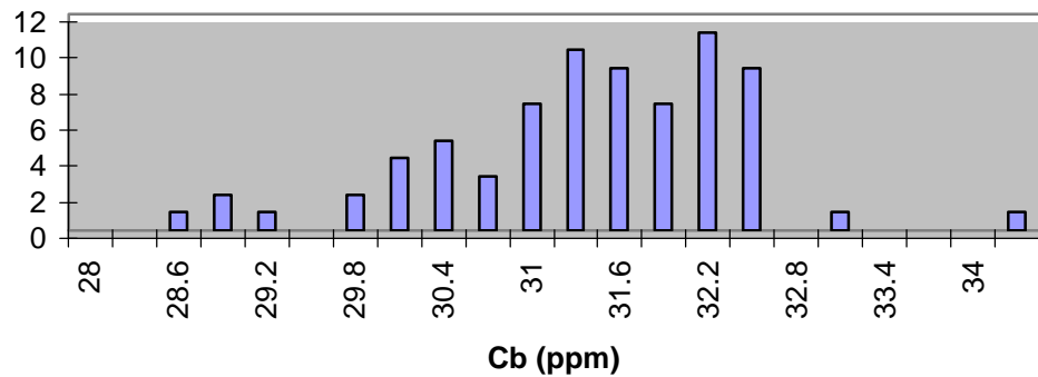
HH P Cb
