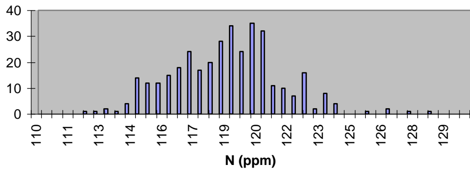
HH Q Ha
