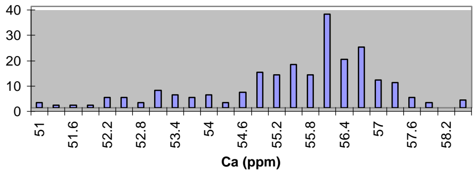
HH N Cb
