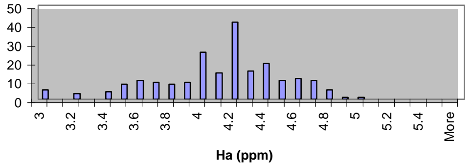
HH M CO
