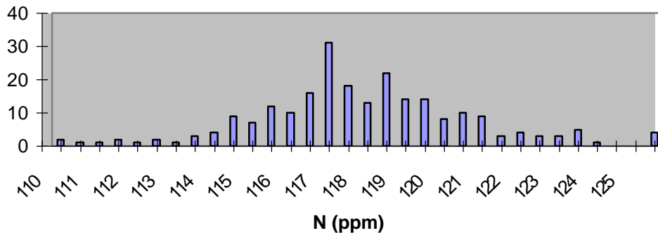
HH N Ha
