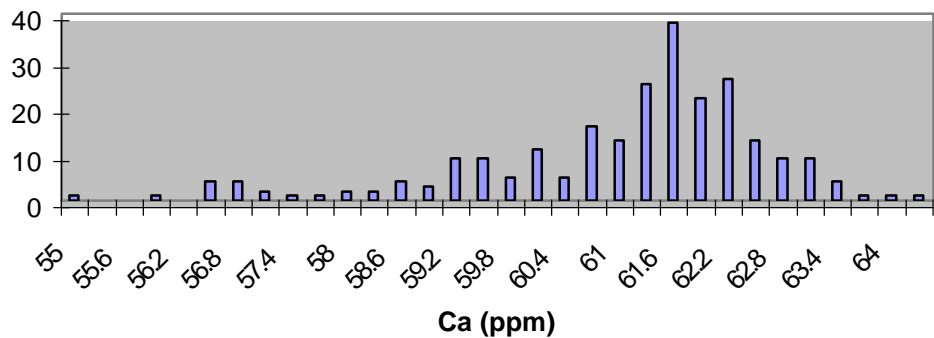
HH S Cb
