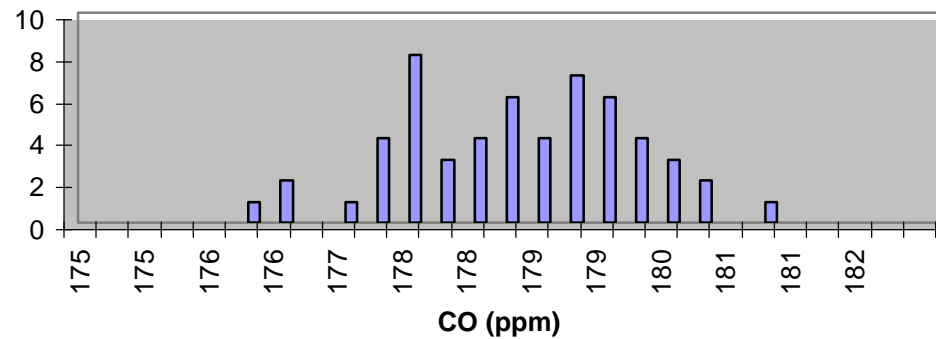
HH P CO
