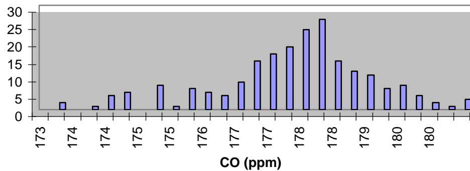
HH V CO
