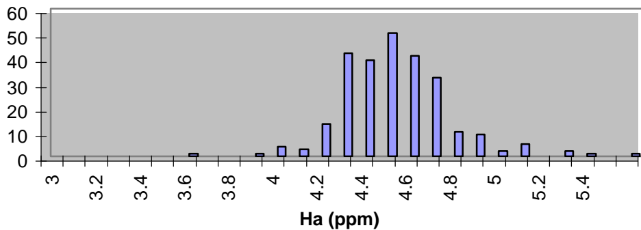
HH N CO
