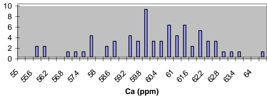
HH W cb
