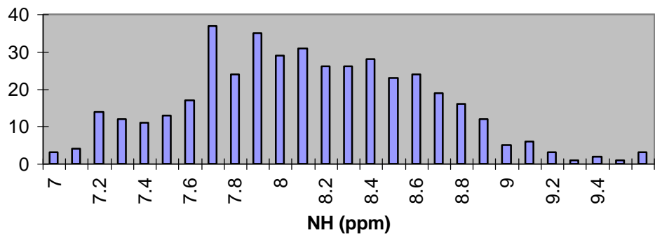
HH Q Ca
