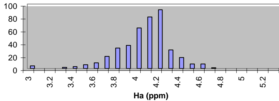
HH Q CO
