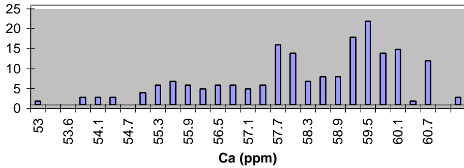
HH M Cb
