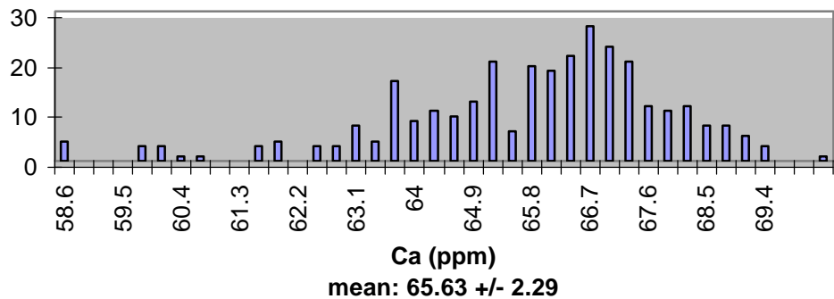
HH T Cb
