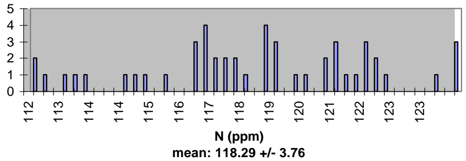
Alpha Helix B Ha
