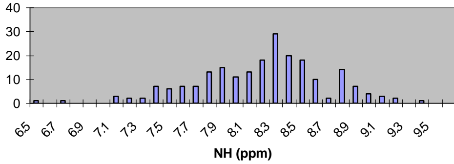
HH M Ca
