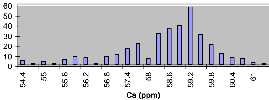
HH Q Cb
