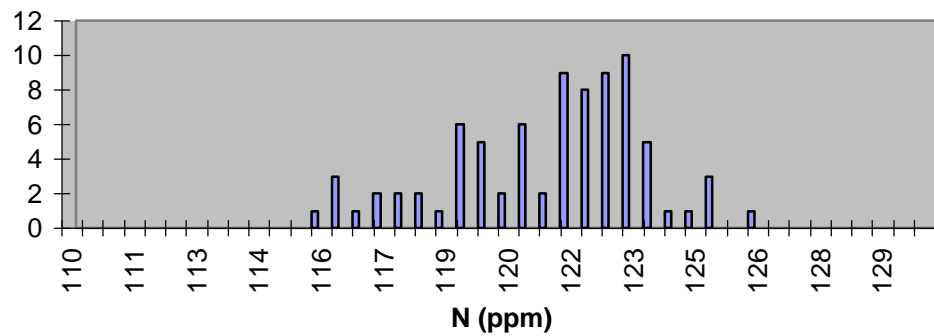
HH W Ha
