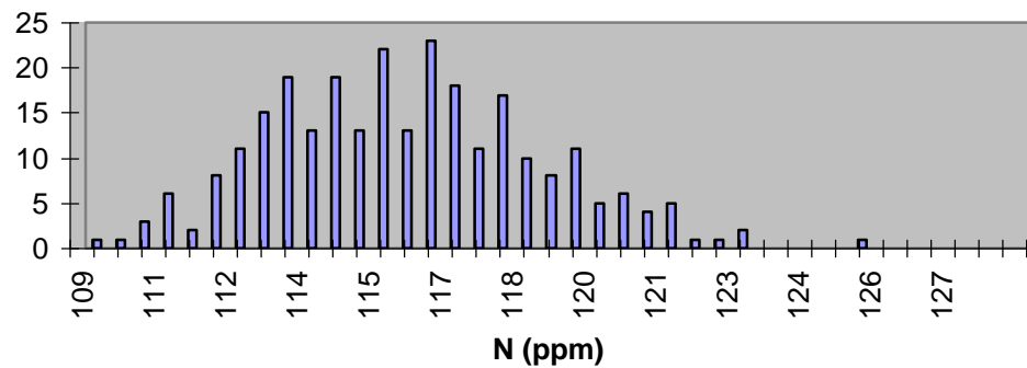
HH S Ha
