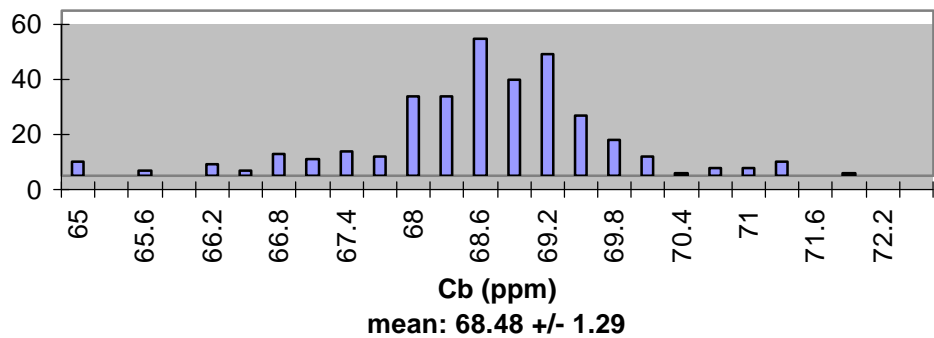
HH T Cb
