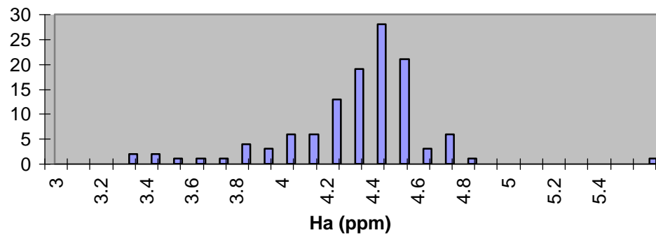
HH P CO
