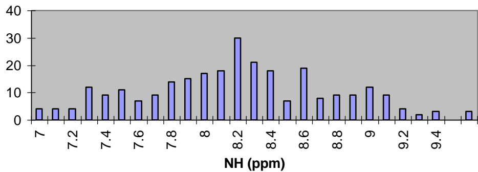
HH Y Ca
