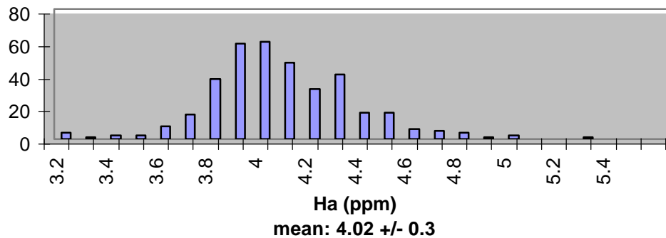
HH T CO
